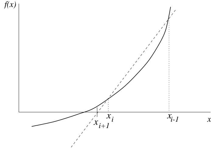
Abbildung 6.5: Sekanten-Verfahren
